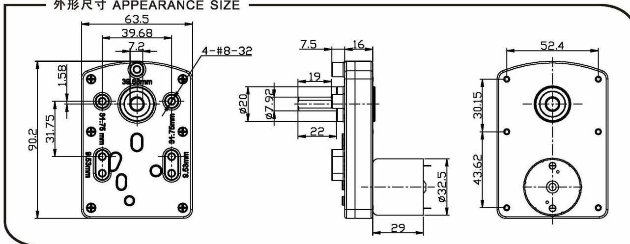
齿轮箱数据 Gearbox data
