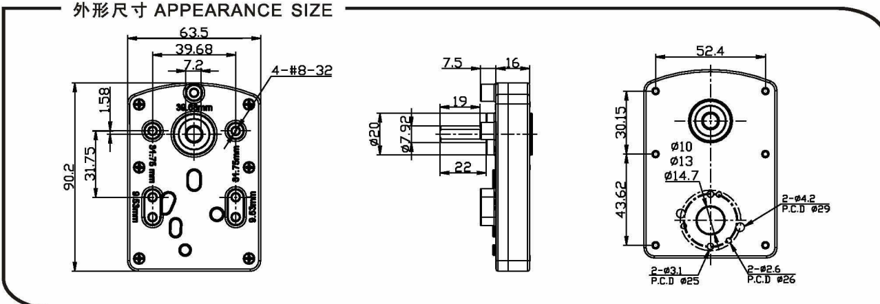
外形尺寸 APPEARANCE SIZE
